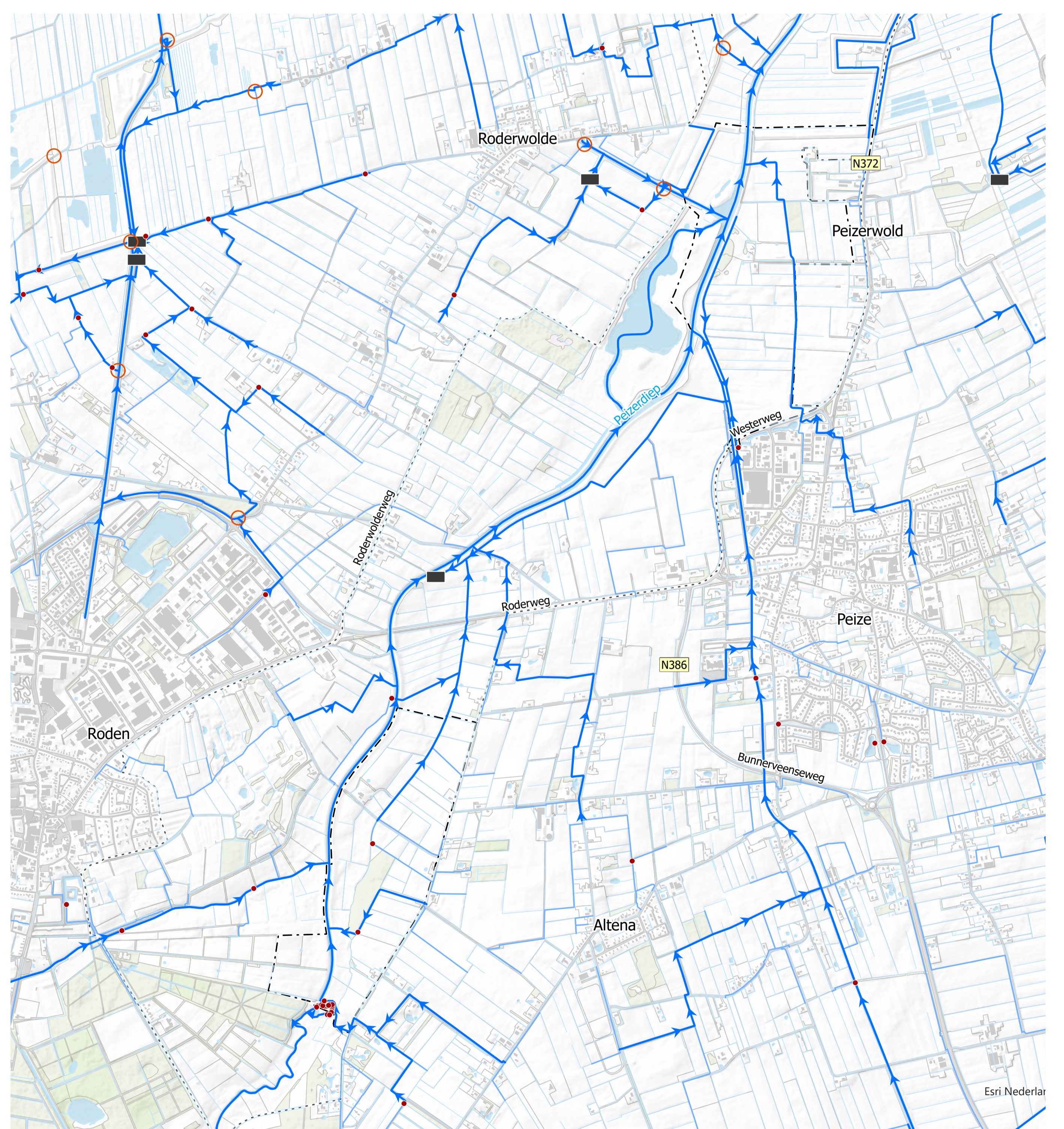
Op snelle afvoer gericht watersysteem
